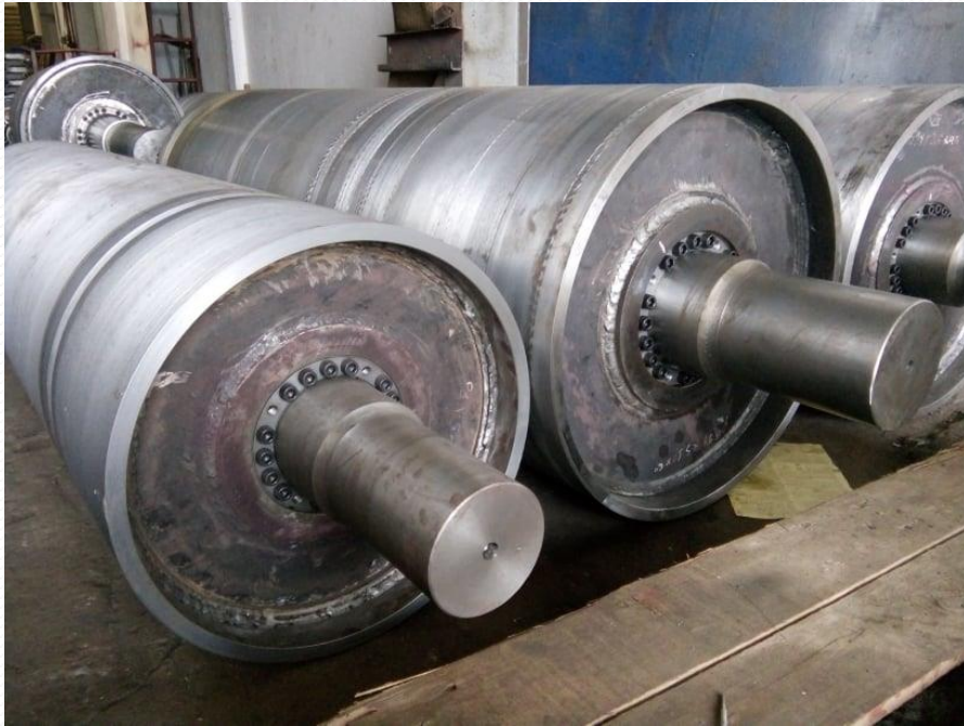
Tang băng tải
